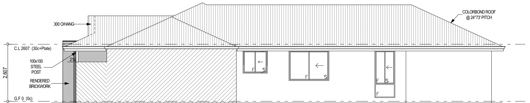
4 ELEVATION 1:100
