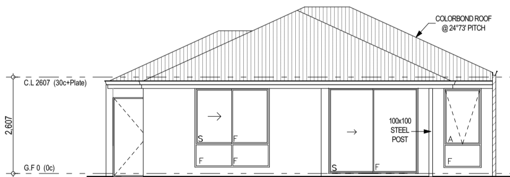
3 ELEVATION 1:100
